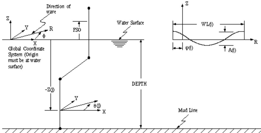
تصویر ۳ مشخصات مصالح Water Table در المان PIPE 59
